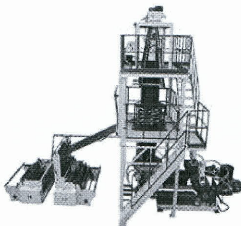
Máy thổi màng hai lớp LDPE
