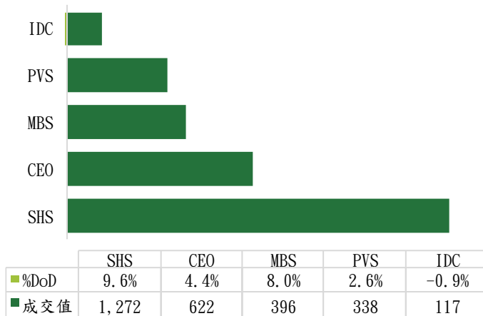
前五大撮合（十億越盾）- HNX指數
