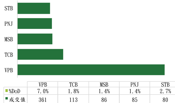
前五名議價（十億越盾）- VN指數
