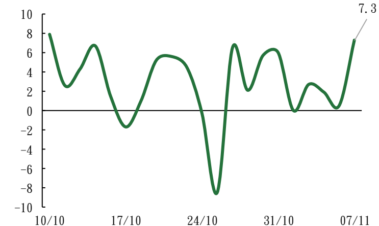
VN30F1M - VN30F2M
