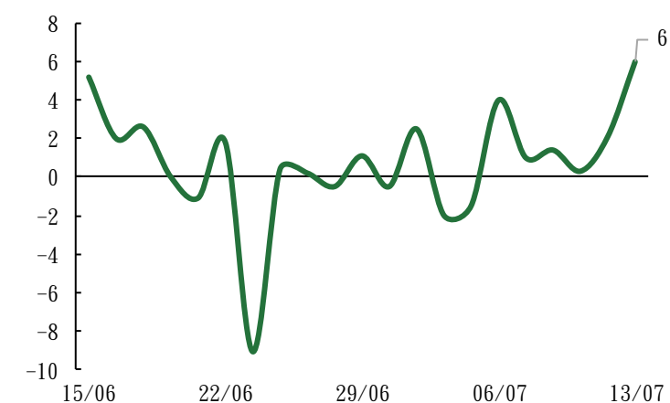
VN30F1M - VN30F2M
